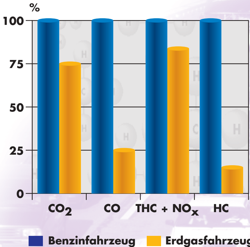
Vergleichsfahrzeug Benzin (100%)
