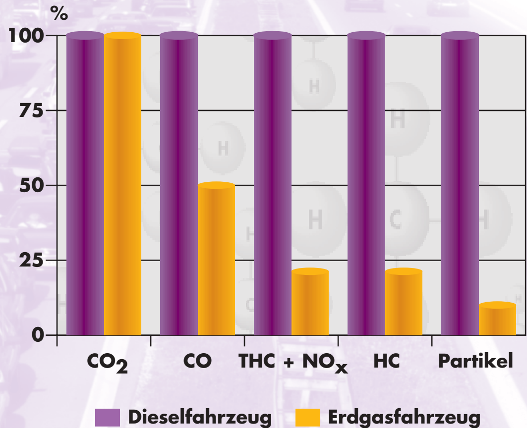
Vergleichsfahrzeug Diesel (100%)
